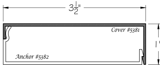
1" x 3 1/2" (D)
