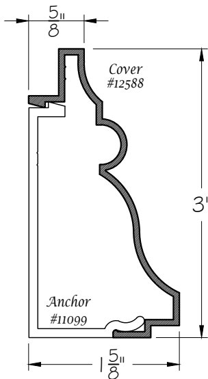
BrickMold (Q)
