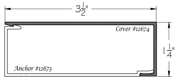
3 1/2" x 1 1/4" (AA)
