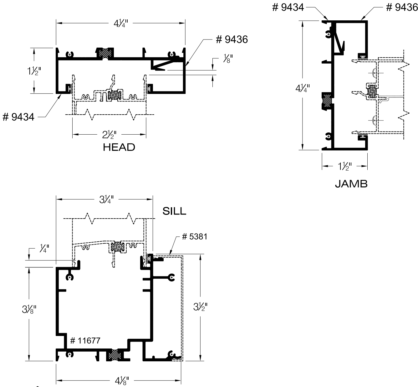
14# Framemaster Subsill
