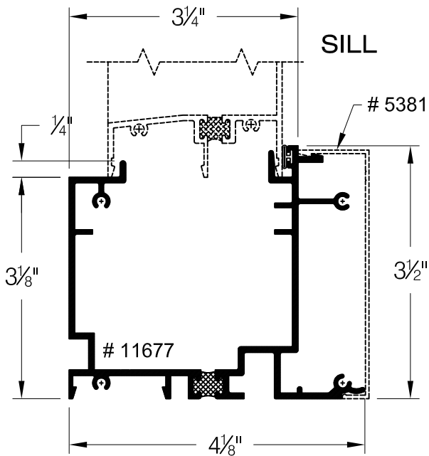
14# Framemaster Subsill
